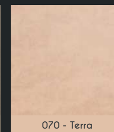
080 - Deserto
